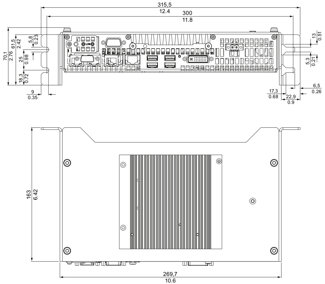
Bild 15-5 Maßbilder des Geräts mit Buchmontagewinkel
