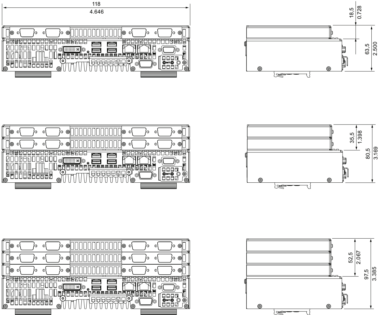
Bild 15-6 Maßbilder des Geräts mit Erweiterungsrahmen
