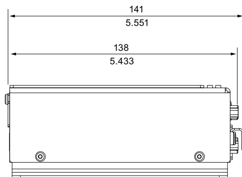
Bild 15-4 Maßbild des Geräts mit Befestigungswinkeln: Seitenansicht
