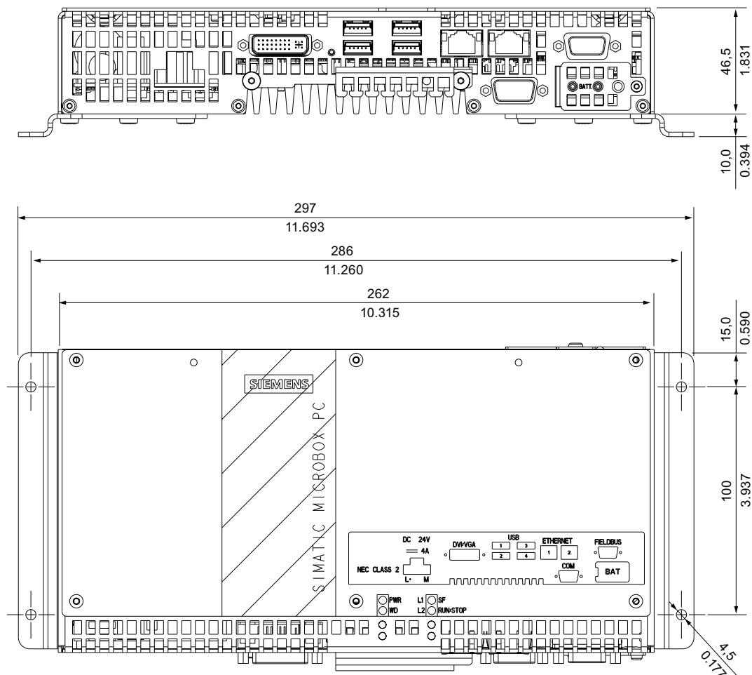
Bild 15-3 Maßbild des Geräts mit Befestigungswinkeln: Vorderansicht und Draufsicht
