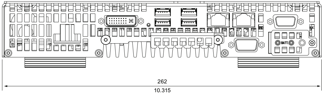
Bild 15-1 Maßbild des Geräts: Vorderansicht
