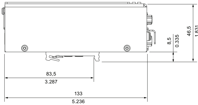
Bild 15-2 Maßbild des Geräts: Seitenansicht
