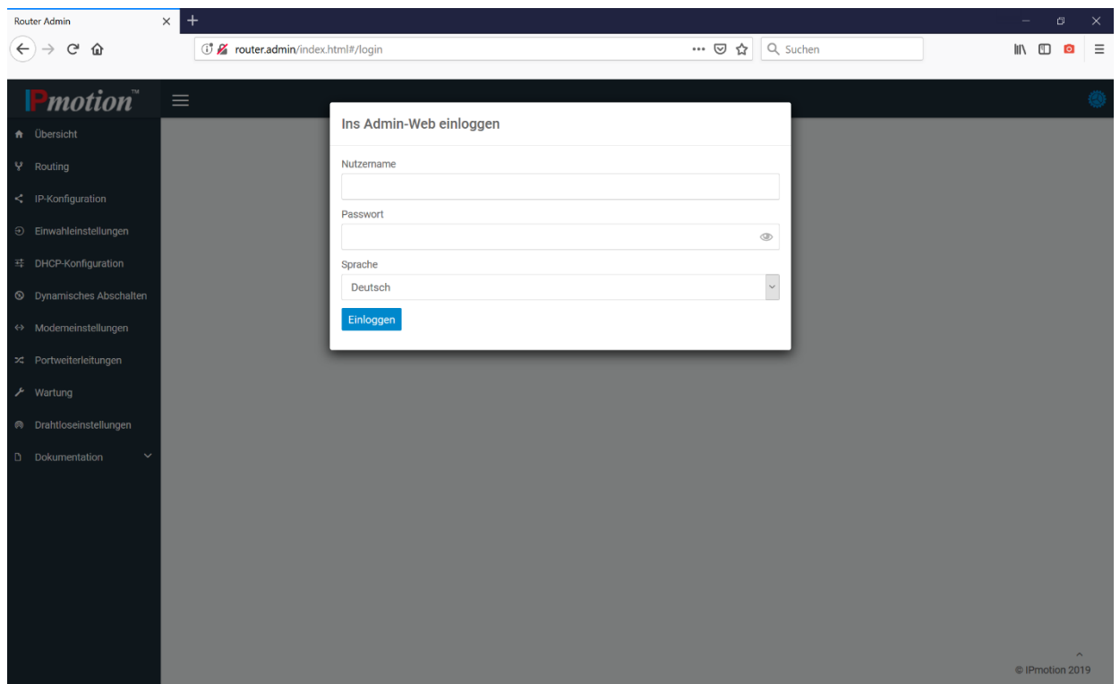
Abb. 5: Einloggen Admin-Web
